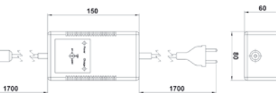
Зарядное устройство HML-ISO 35
